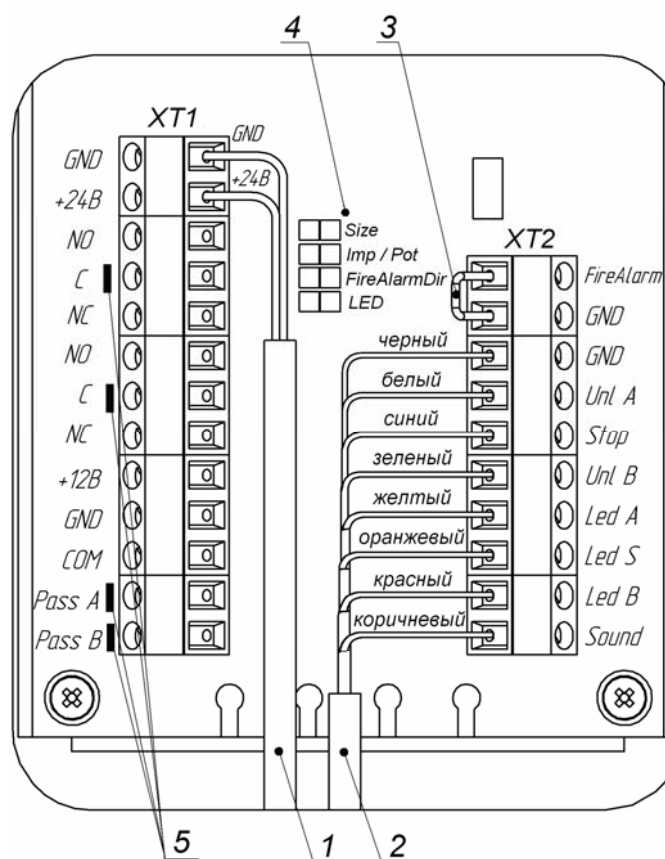
Рисунок 3. Внешний вид платы управления
