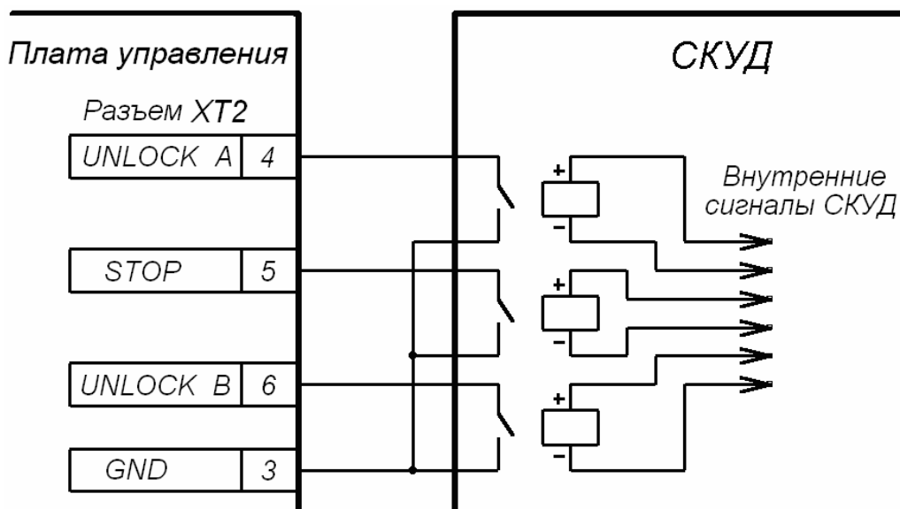
Рисунок 6. Управляющий элемент СКУД нормально разомкнутый контакт реле
