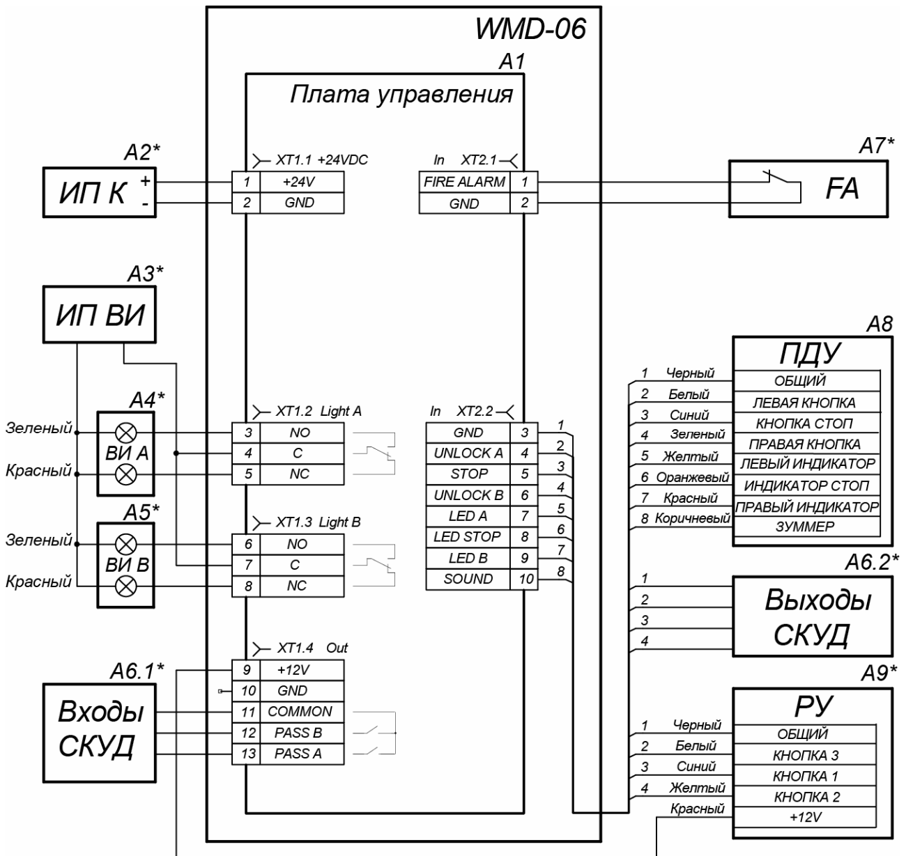
Рисунок 11. Схема электрических соединений
