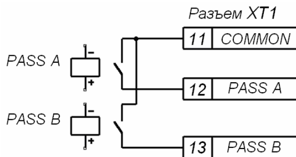
Рисунок 8. Выходные каскады для PASS A , PASS B
