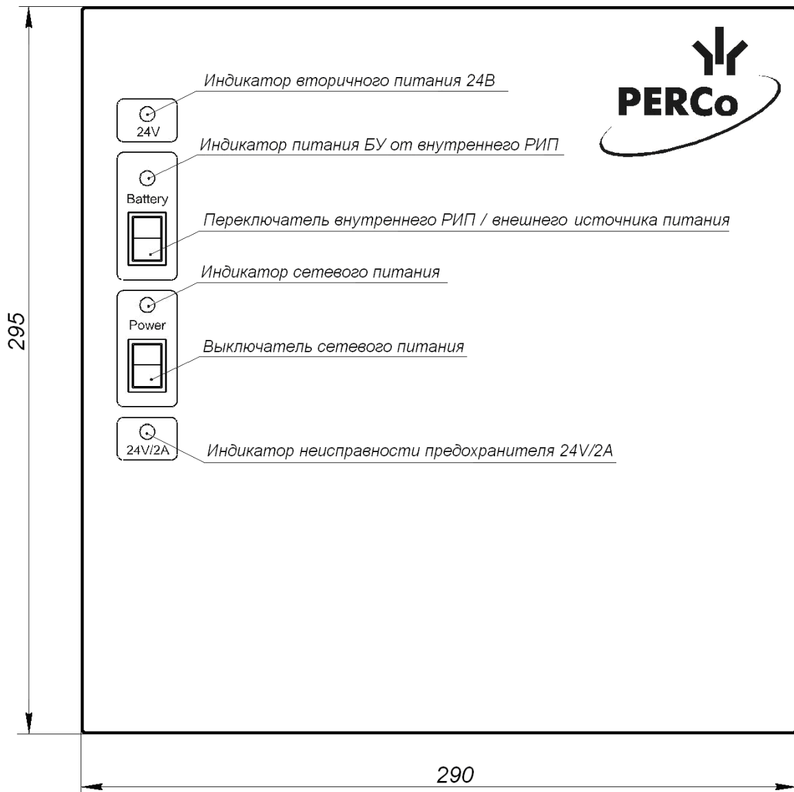
Рисунок 3 Блок управления
