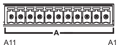
Гнезда разъемного соединителя сигнализации и контроля ALARM/CONTROL A
