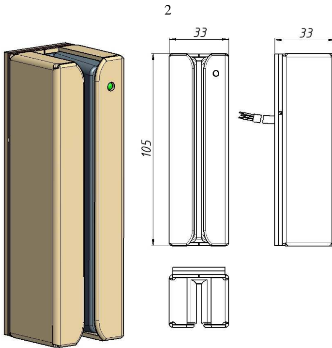
Рис.1 Считыватель
