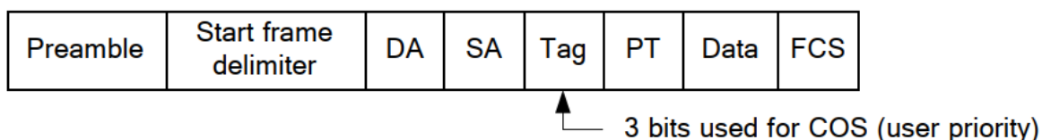
Рисунок 2-14. Приоритеты класса сервиса (CoS)
