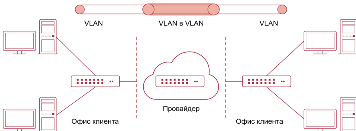
Рисунок 2-4. QinQ
