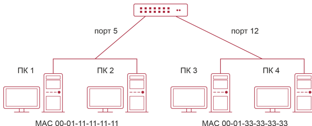
Рисунок 2-13. Динамическое построение таблицы MAC-адресов
