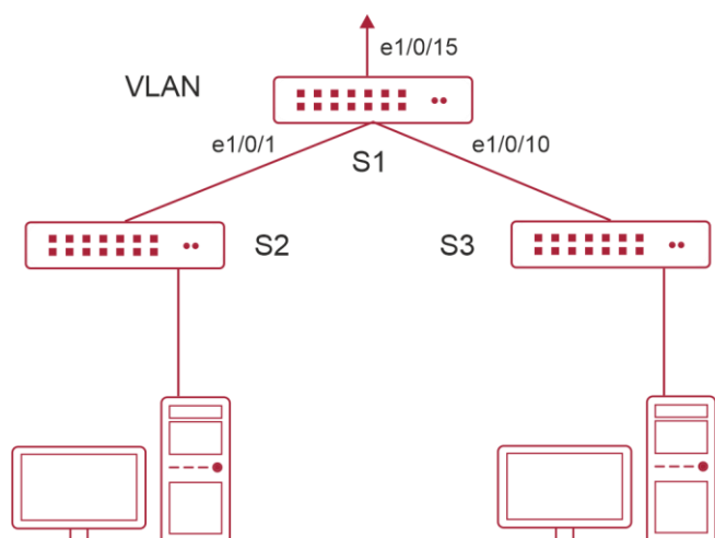
Рисунок 2-7. Типовые примеры функции изоляции портов
