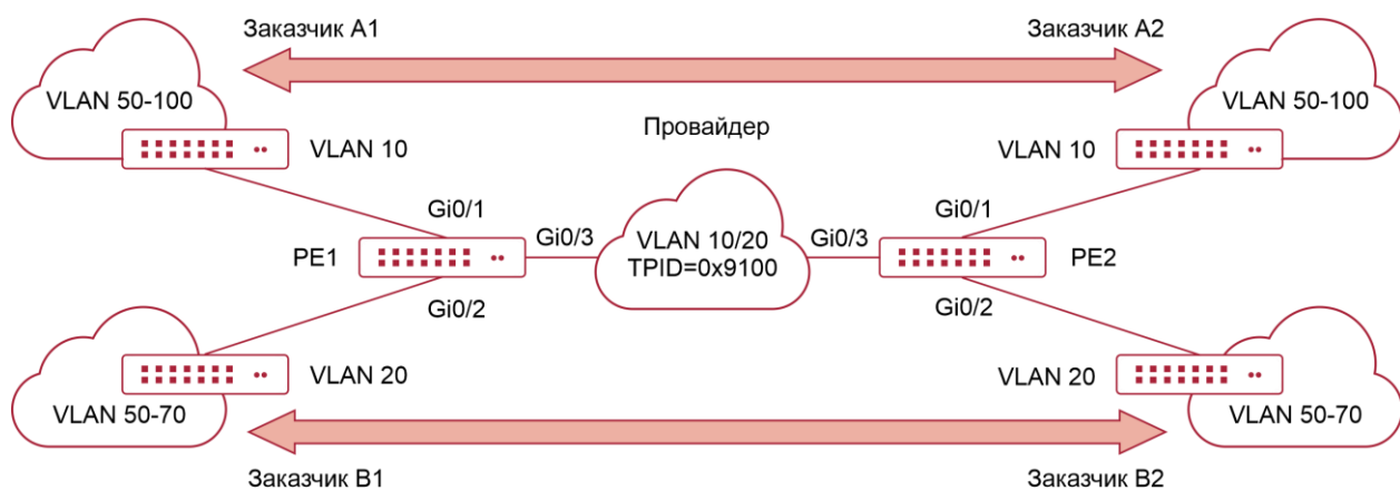
Рисунок 2-5. Port-based QinQ
