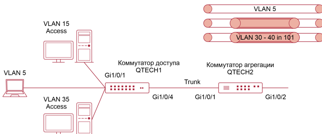
Рисунок 2-6. Selective QinQ
