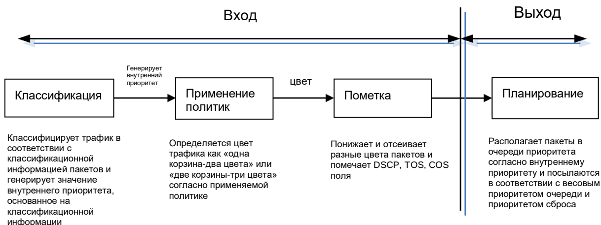
Рисунок 2-17. Базовая модель QoS
