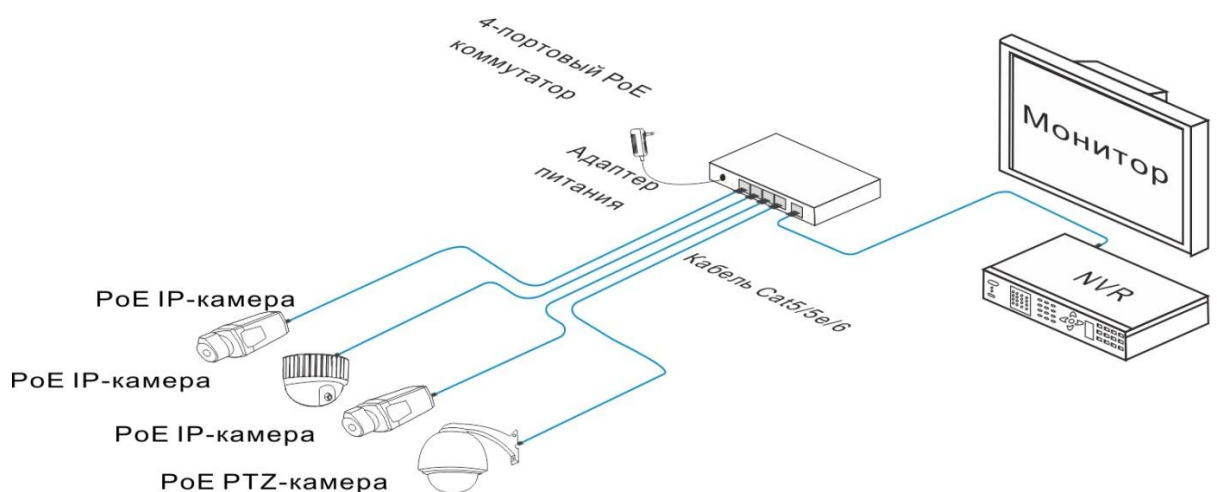
Рис. 5 Общая схема подключения
