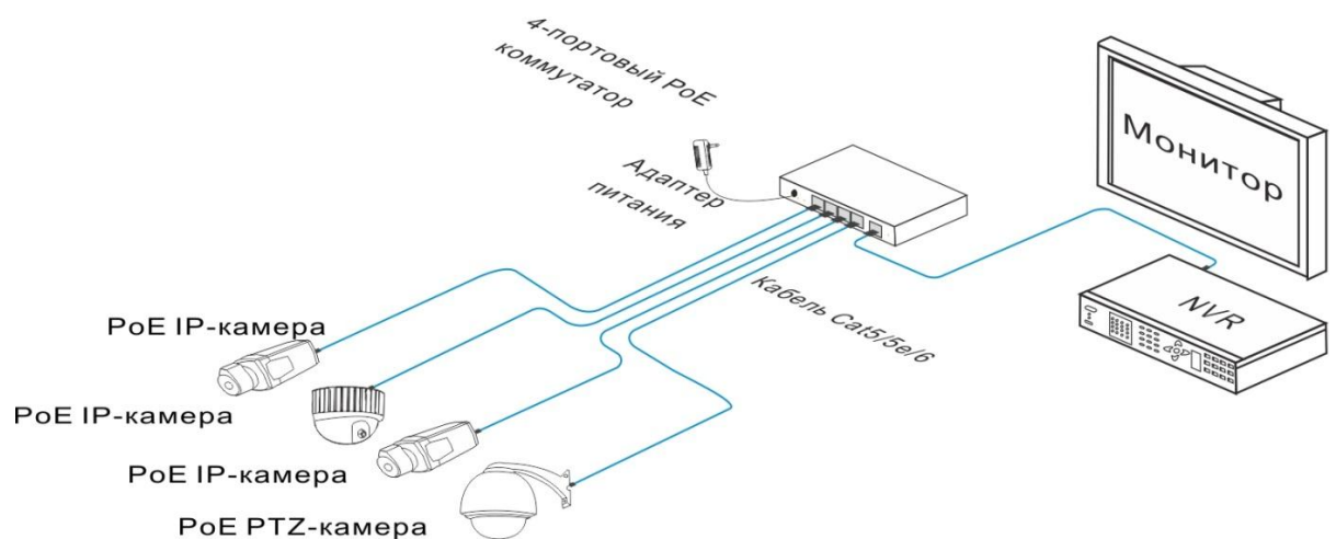
Мал. 2 Агульная схема падключэння
