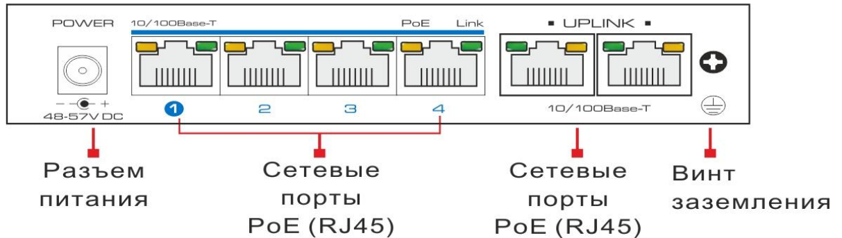
Рис. 1 Задняя панель коммутатора
