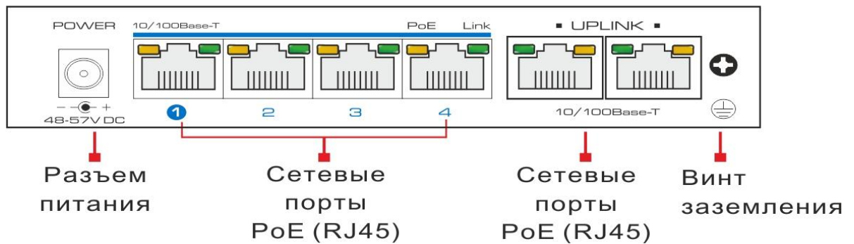
Мал. 1 Задня панель комутатора
