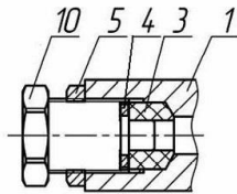
ЗГ, заглушка для отверстия под кабельный ввод
