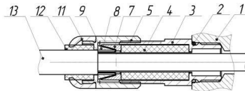
КВ-БК-12 – монтаж бронированным кабелем
