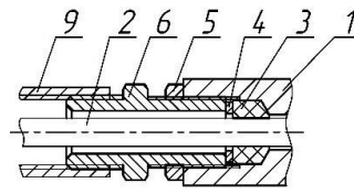
ШТ, для монтажа кабелем в металлической трубе
