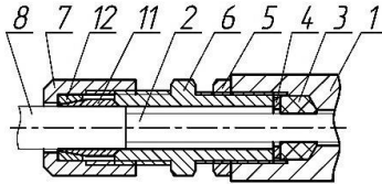
КВ-12, для монтажа кабелем в металлорукаве или бронированном кабелем
