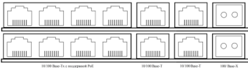
Рисунок 3. Коммутационная панель коммутатора Релион-SW-Exd-A/H-8-PoE/ PoE+
