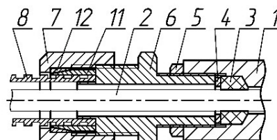
монтаж кабелем в металлорукаве KV15, KV18, KV20
