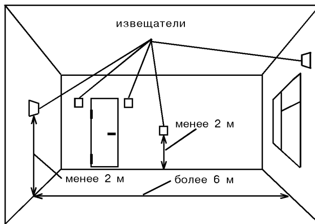
Рис. 10 - Не рекомендуемые места установки извещателя
