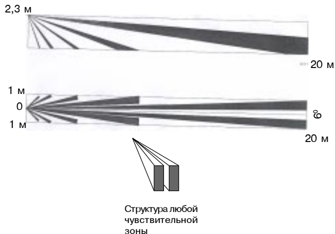
Рис. 1. Диаграмма зоны обнаружения
