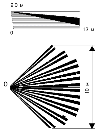
Рис. 1 – Диаграмма зоны обнаружения
