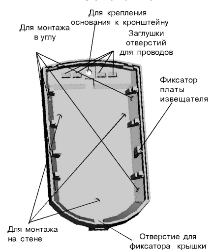
Рис. 1. Основание извещателя и кронштейн
