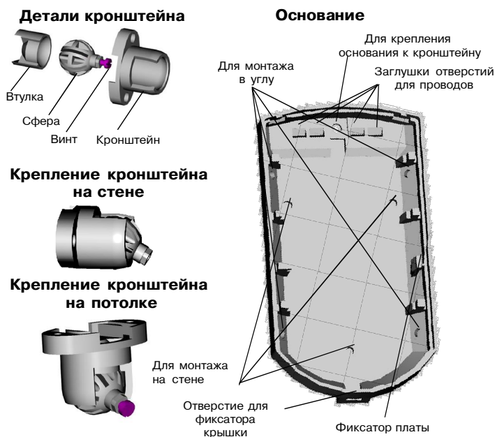
Рис. 2. Основание извещателя и кронштейн
