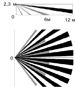
Рис. 1. Диаграмма зоны обнаружения
