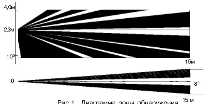
Рис.1 Диаграмма зоны обнаружения 15 м
