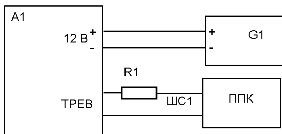
Рис.1 Схема подключения извещателя
