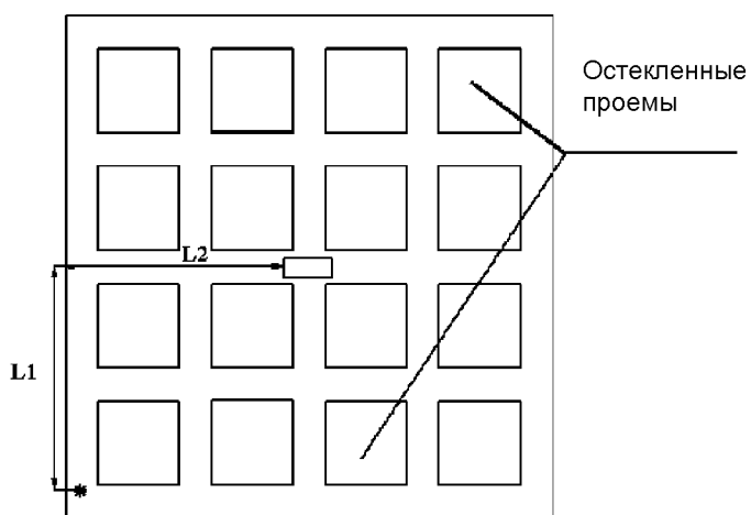
Рис.5 Защита переплета оконной рамы
