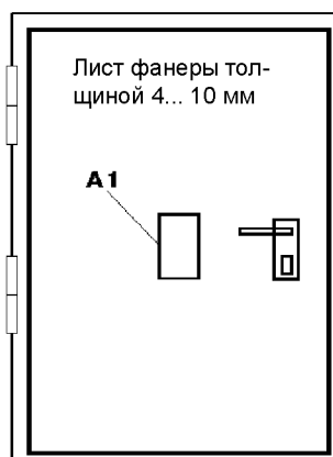
Рис.9 Защита деревянной пустотелой двери
