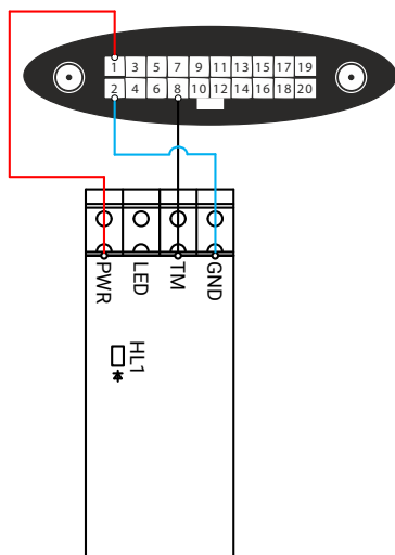
Рисунок 72. Схема подключения считывателя MIF
