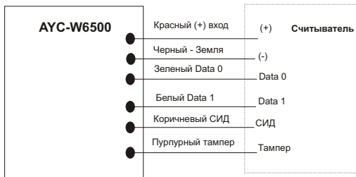
Рисунок 5: Подключение считывателя
