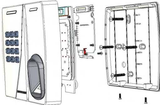
Рисунок 1 АУС-W6500 установка
