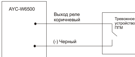
Рисунок #3 Подключение тревожного устройства
