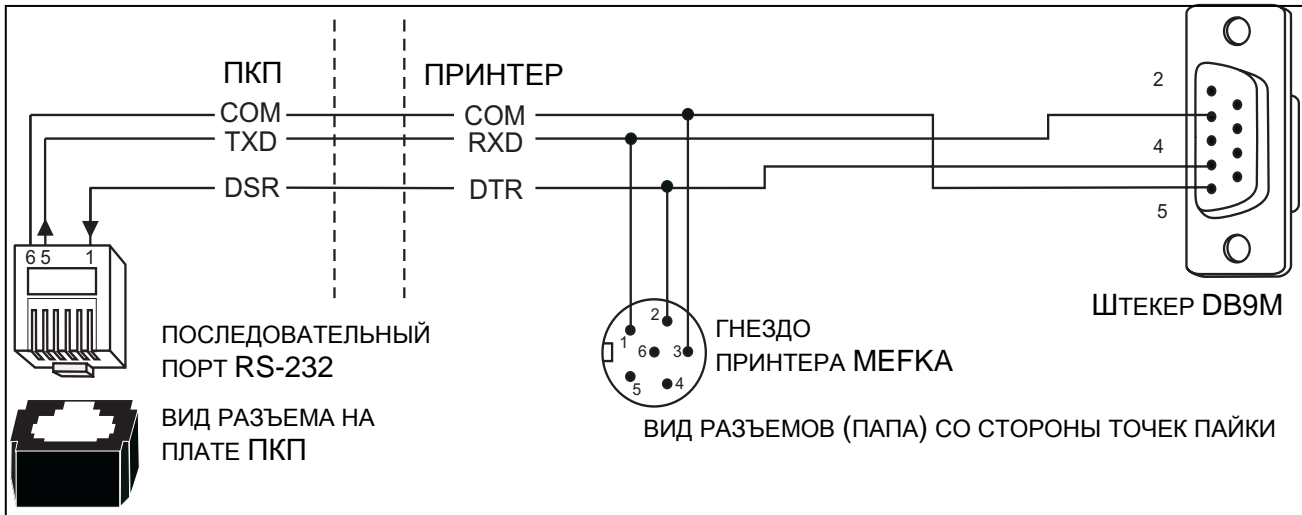
Рис. 16. Способ подключения принтера к порту RS-232 ПКП.
