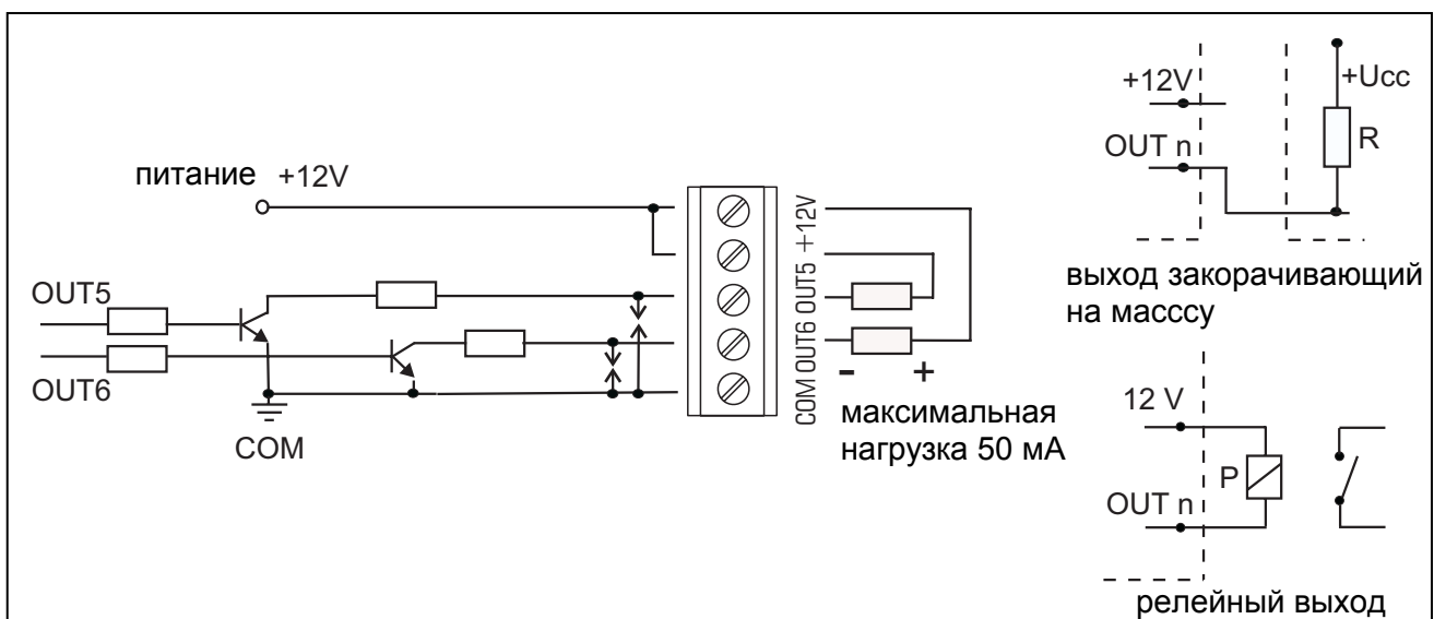
Рис. 13. Схема слаботочных выходов OUT5 и OUT6 и подключение нагрузки.
