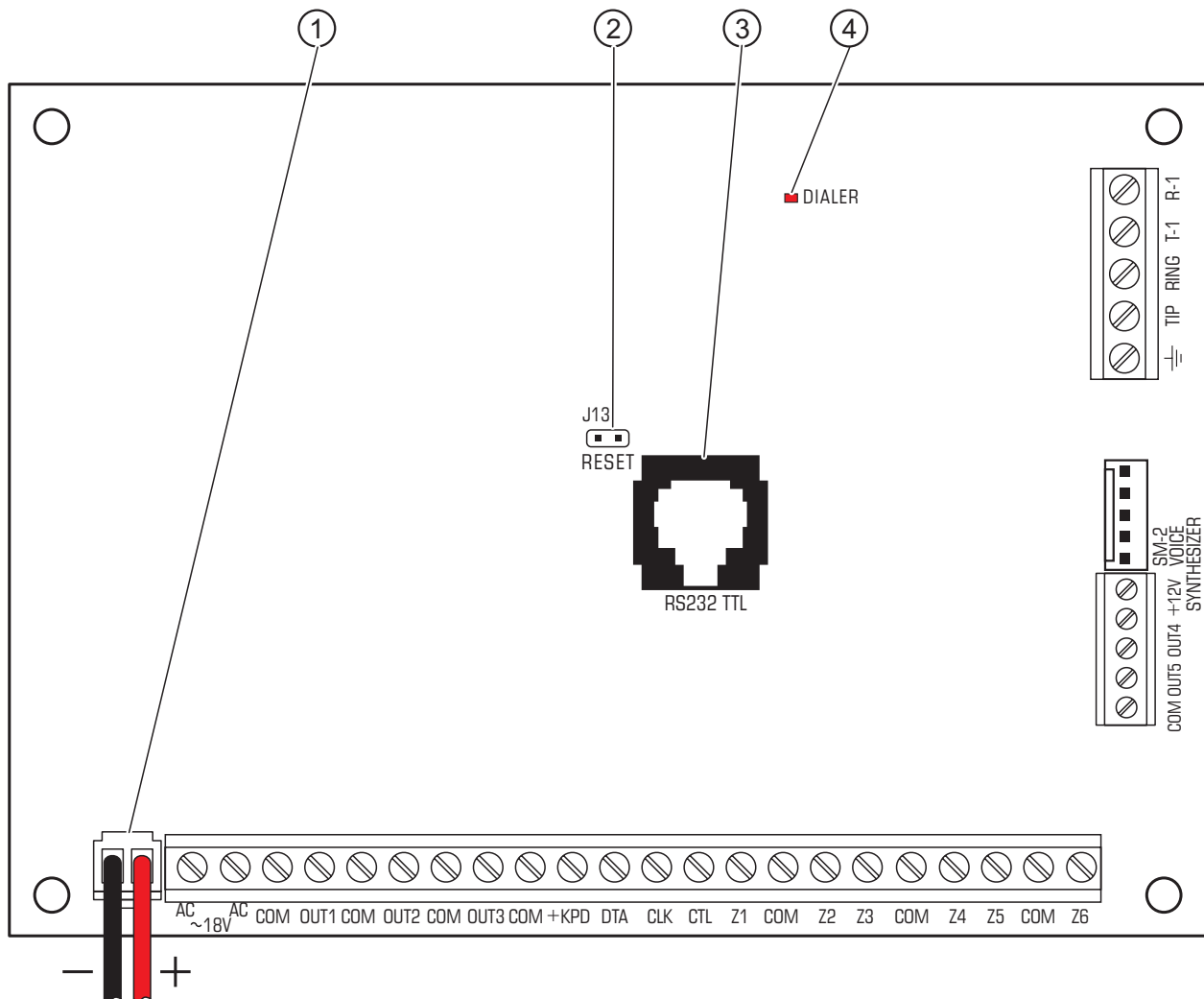
Рисунок 2. Вид платы ПКП CA-6
