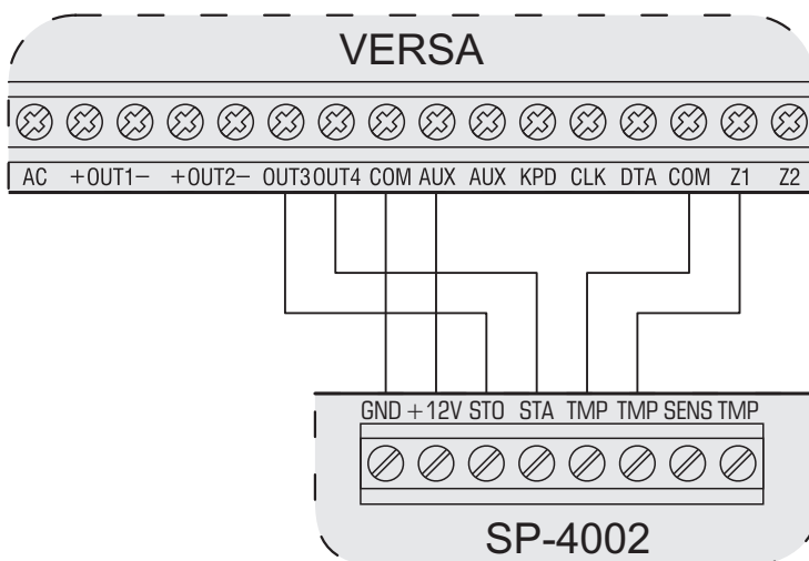
Рис. 26. Способ подключения к слаботочным выходам ПКП оповещателя с собственным питанием (на примере SP-4002).
