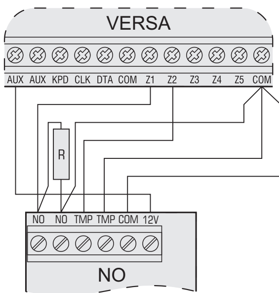
Рис. 22. Пример подключения к ПКП извещателя NO по схеме EOL.
