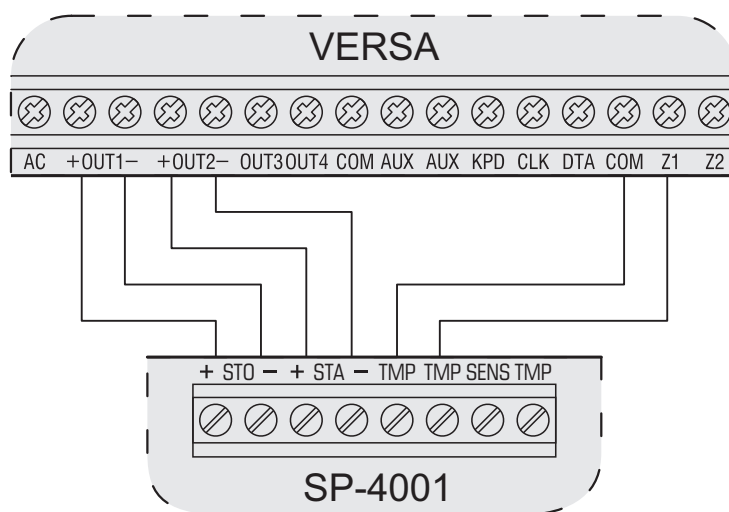
Рис. 25. Способ подключения к силовым выходам ПКП оповещателя без собственного питания (на примере SP-4001).
