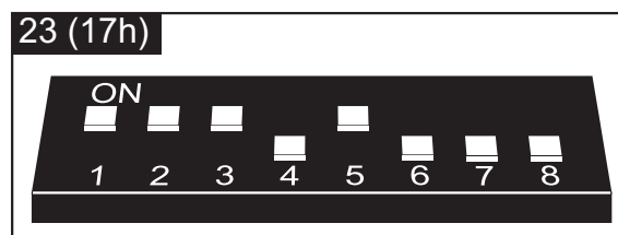
Рис. 20. Способ установки адреса в модуле CA-64 SM. 8 переключатель установлен в положение OFF, т.е. функция записи голосовых сообщений заблокирована.
