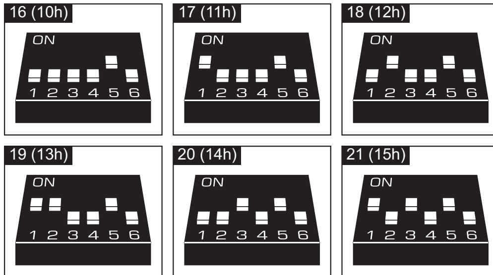
Рис. 19. Способ установки адресов в считывателях INT-IT.
