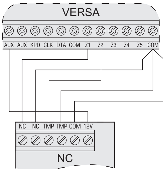
Рис. 21. Пример подключения к ПКП извещателя NC (извещатель NO подключается идентично).
