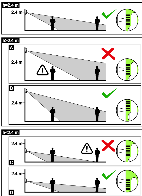
Рис. 7. Влияние высоты монтажа на охраняемую площадь и способ позиционирования пирозлемента по отношению к линзе с целью оптимальной установки. В зависимости от высоты монтажа средний штрих шкалы должен находиться напротив отметки на корпусе (монтаж на высоте 2,4 м), выше отметки (монтаж выше 2,4 м – пример В) или ниже отметки (монтаж ниже 2,4 м – пример D).
