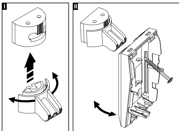
Рис. 6. Монтаж извещателя на кронштейне.
