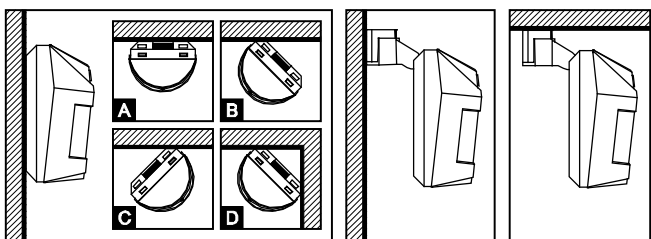
Рис. 5. Способ монтажа извещателя.
