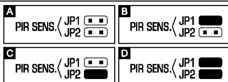
Рис. 2. Способ установки чувствительности извещателя (А – низкая чувствительность, В и С – средняя чувствительность, D - высокая чувствительность)
