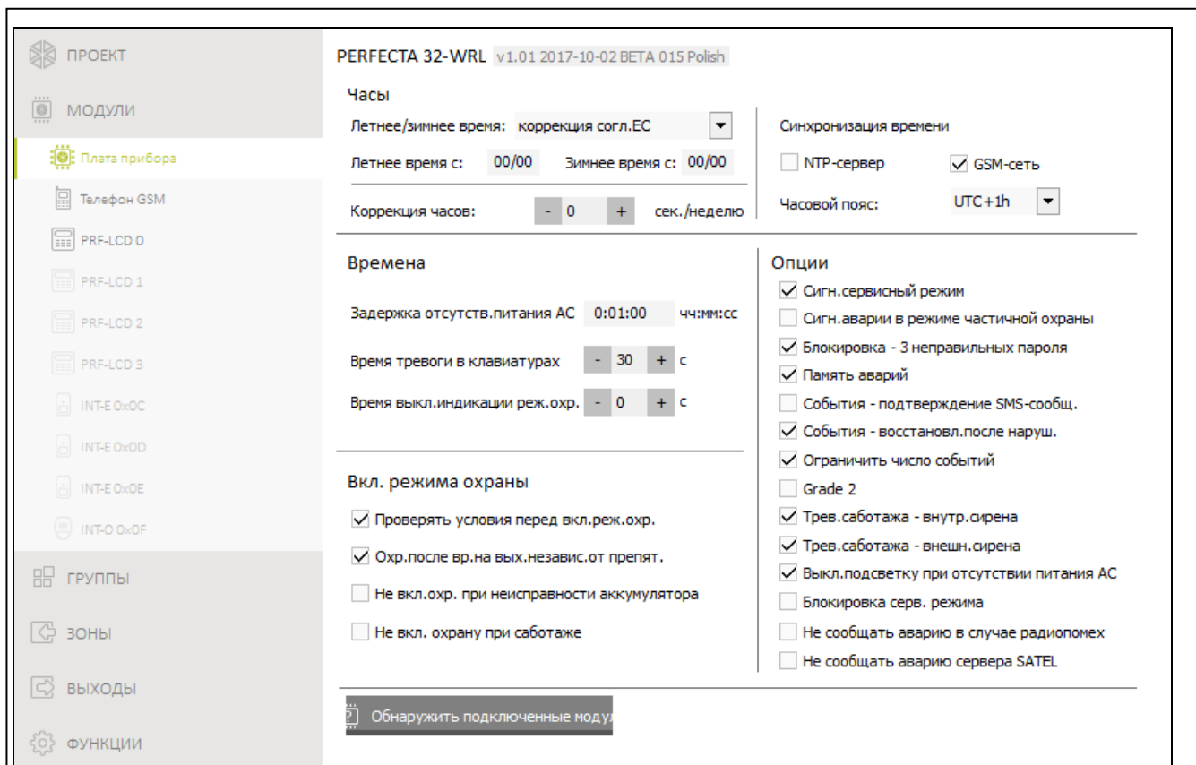
Рис. 8. Закладка "Плата прибора".
