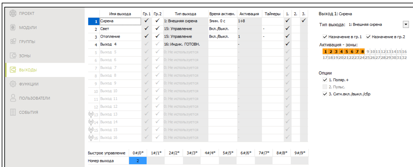
Рис. 16. Закладка "Выходы".
