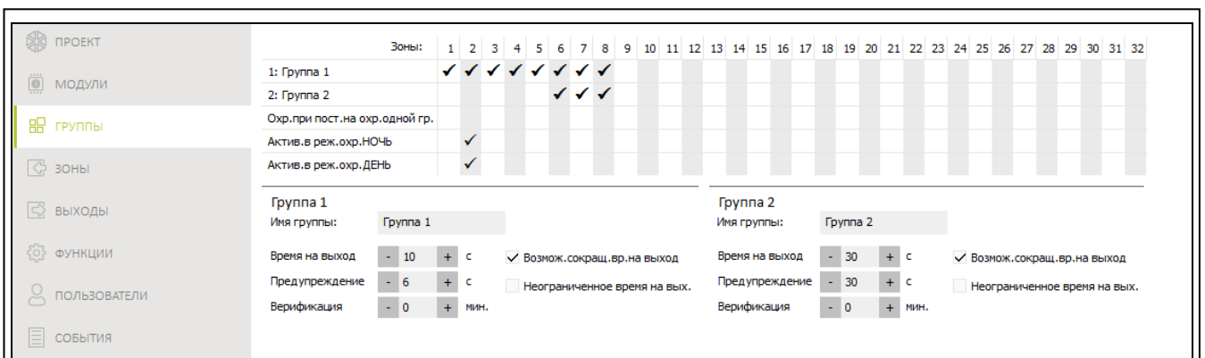
Рис. 14. Закладка "Зоны доступа".
