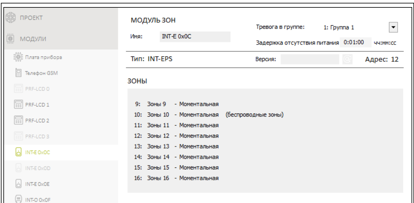
Рис. 12. Закладка с установками модуля расширения зон.
