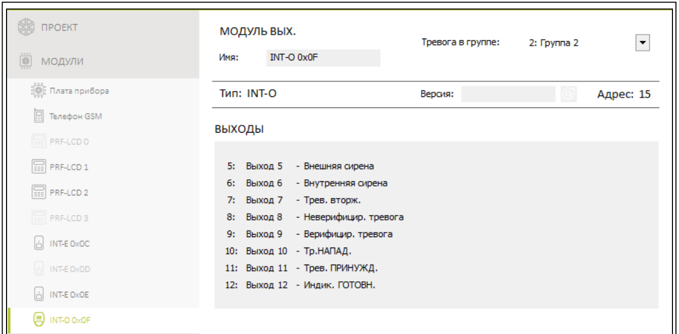
Рис. 13. Закладка с установками модуля расширения выходов.
