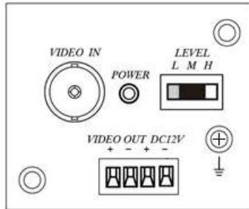
Рис.2 Панель подключения ТТА111ТВIT
