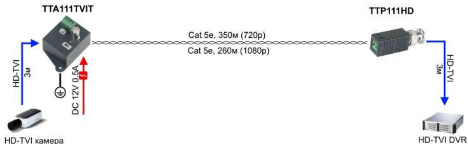
Рис.3 Схема подключения TTA111TVIT
