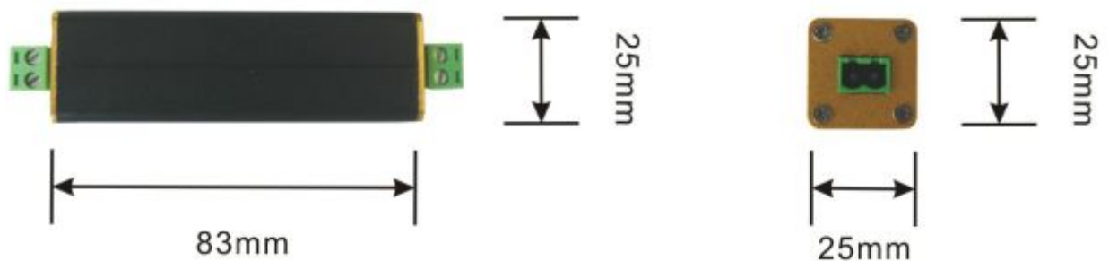
Рис.2 Габаритные размеры SP-IP/100
