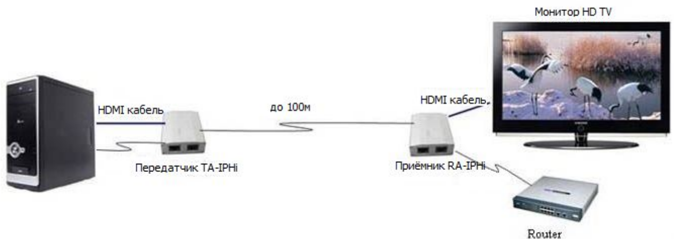
Рис.4 Схема подключения передатчика TA-IPHi и приемника RA-IPHi
