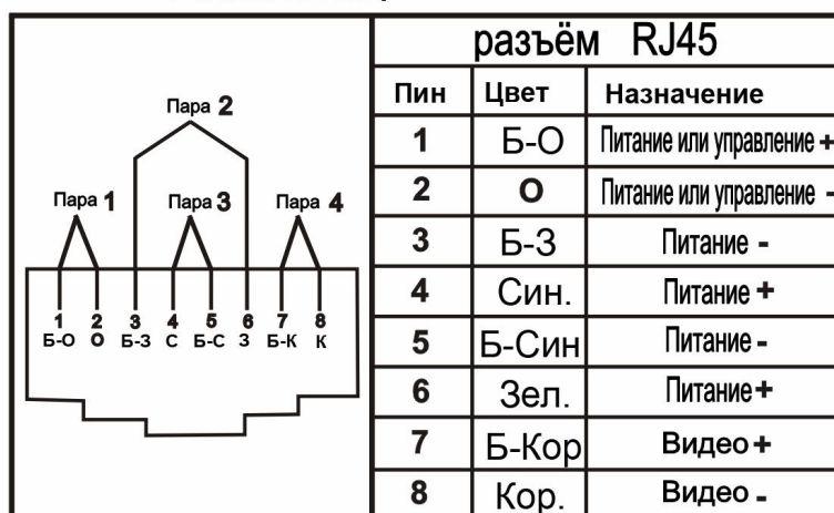
Рис.3 Распиновка разъёма RJ45
