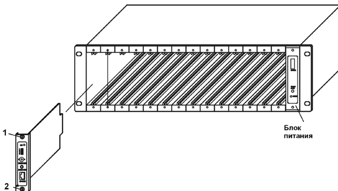
Рис. 2 Монтаж устройств в бокс TRN012
