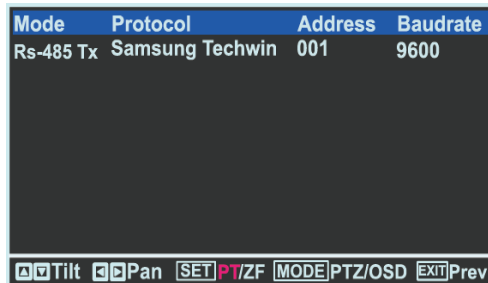
Рис.9 Экран режима RS485 Tx
