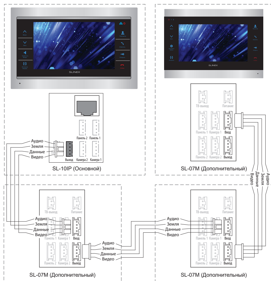
Схема 2. Подключение системы домофонов SL-10IP и SL-07M.
