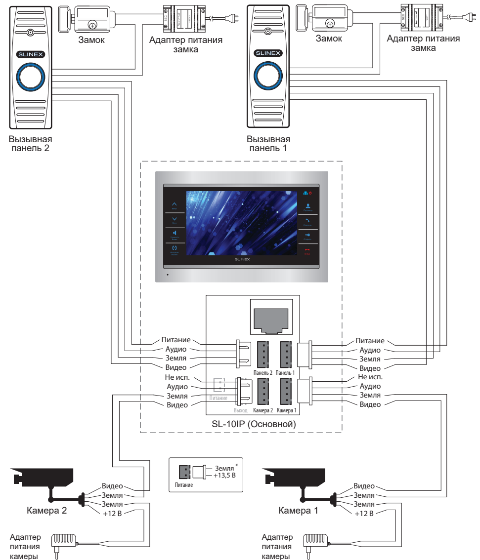
Схема 1. Подключение вызывных панелей и камер к домофону SL-10IP.
