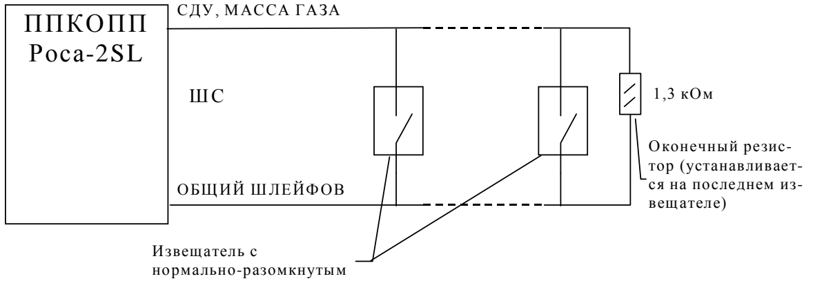
Рисунок 7. Включение извещателей в сигнальные шлейфы.
