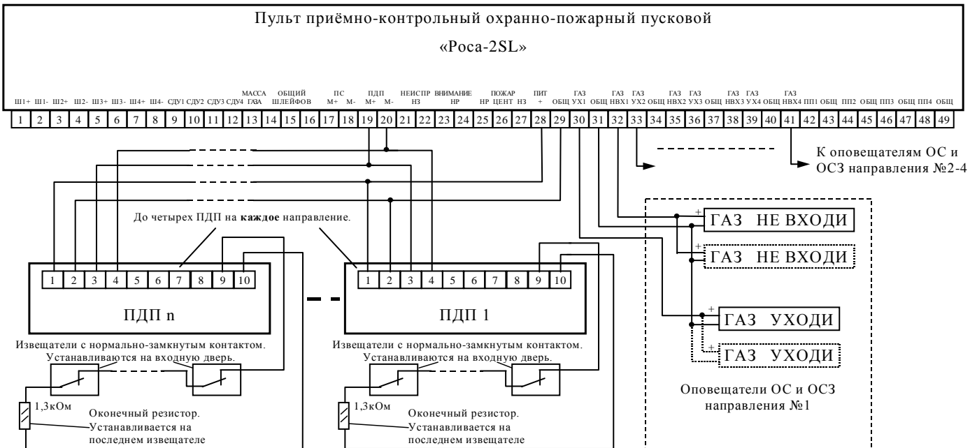
Рисунок 9. Схема подключения БККП к ПКОПП «Роса-2SL».
