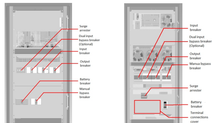
Рис. 3.1.3. Вид спереди с открытой фронтальной крышкой а) Устройства мощностью от 20 до 30 КВА б) Устройства мощностью от 40 до 80 КВА
