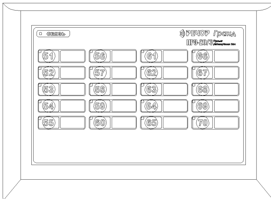
Рис. 3. Лицевая панель пульта расширения зон ПРЗ-20/3.
