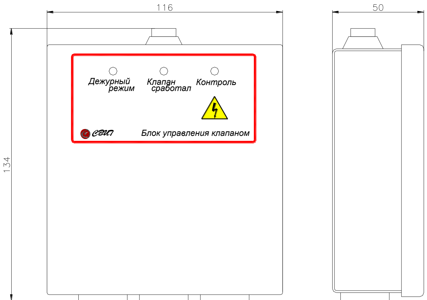
Рис. 2. Внешний вид ВУОК в металлическом корпусе
