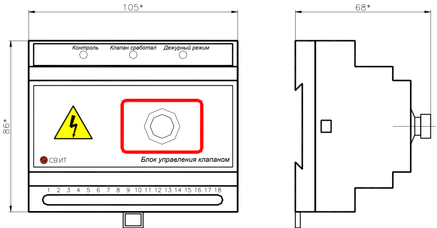
Рис. 1. Внешний вид ВУОК в пластмассовом корпусе
