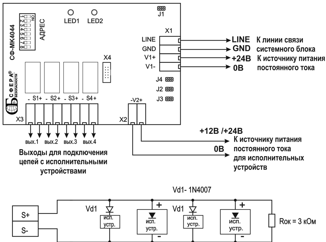
Рисунок 1 Схема внешних подключений «СФ-МК4044».
