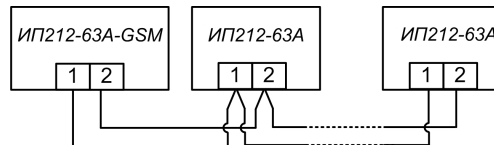
Рисунок 2 – Схема соединения извещателей в группу
