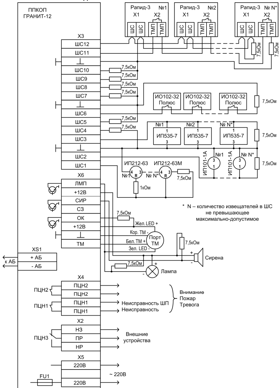
Рис.6 Схема внешних соединения прибора «Гранит-12»
