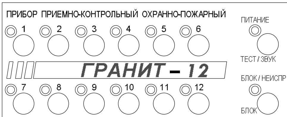
Рис.4 Внешний вид панели индикации и управления прибора «Гранит-12»
