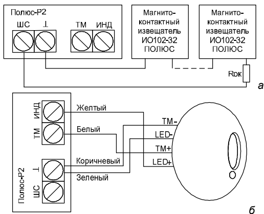
Рисунок 10 – Схемы подключений
