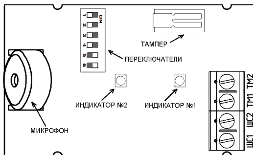
Рис. 1 Плата извещателя
