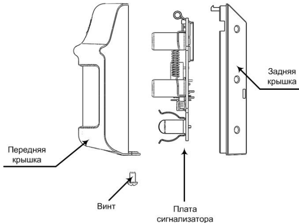
Рис.1 Конструкция сигнализатора
