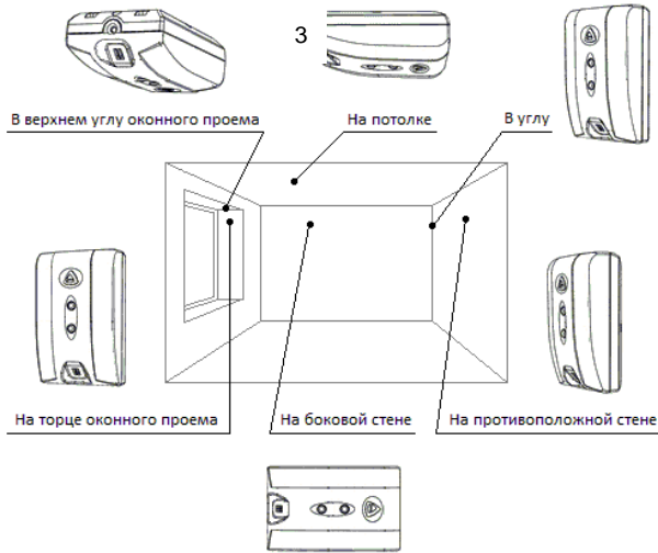
Рис. 2 Возможные варианты установки извещателя
