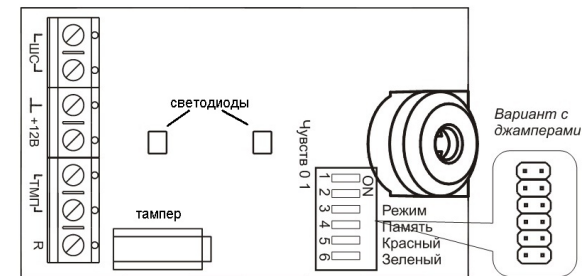
Рис. 1 Плата извещателя
