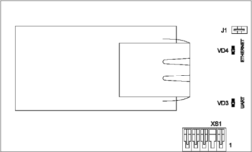
Рис. 12 Внешний вид платы IP-коммуникатора
