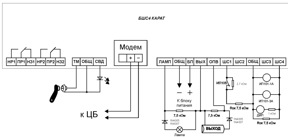
Рис. 7 Схема соединения БШС4 и ЦБ
