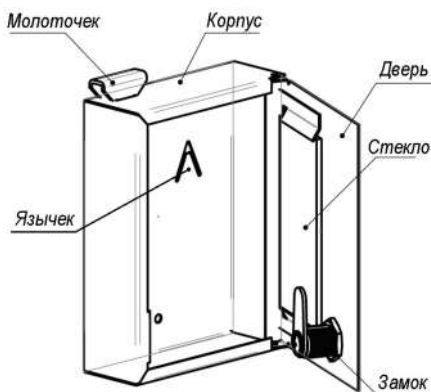
Рисунок 1 – Ключница КЛ-1
