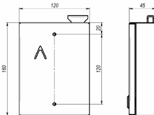
Рисунок 2 – Установочные и присоединительные размеры ключницы КЛ-1
