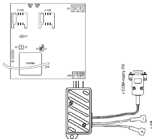
Рис. 2 Подключение адаптера программатора к GT-коммуникатору
