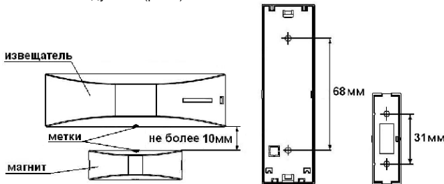
Рис. 1 Общий вид, установочные и присоединительные размеры
