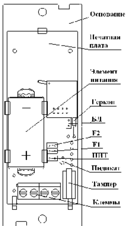
Рис. 13 «ПОЛЮС-Р». Вид изнутри
