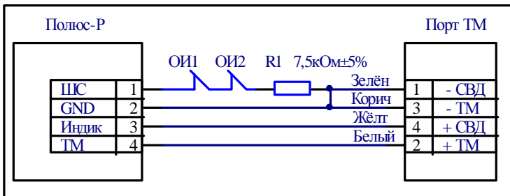
Рис. 14 Подключение шлейфа сигнализации и порта Touch Memory к извещателю «ПОЛЮС-Р»
