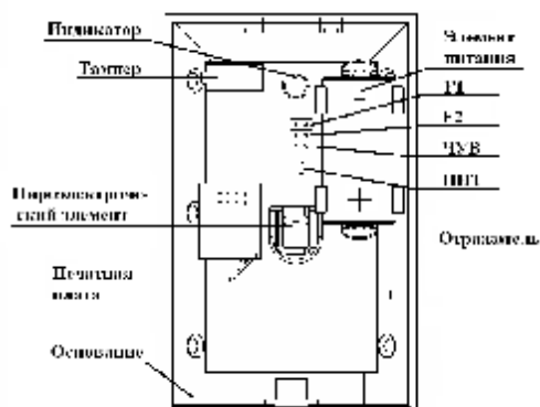
Рис. 12 «РАПИД-Р». Вид изнутри
