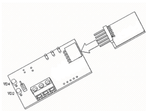
Рис. 11 Соединение основной и дополнительной плат расширения
