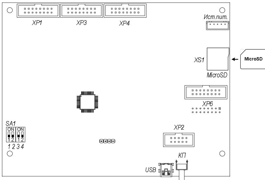
Рис.1 Внешний вид платы контроллера
