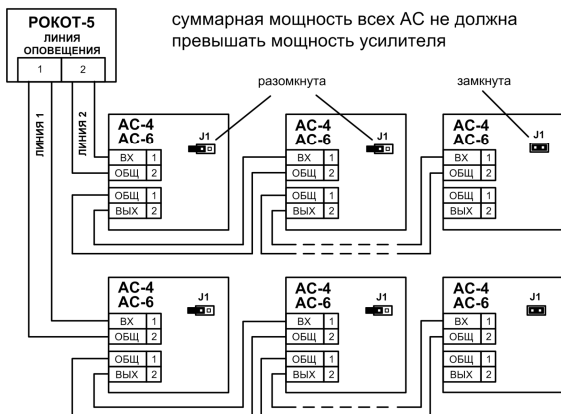
Рис.4 Схема подключений АС-4, АС-6 к линиям оповещения
