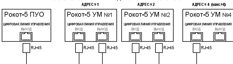
Рис.5 Схема внешних подключений «Рокот-5 УМ»
