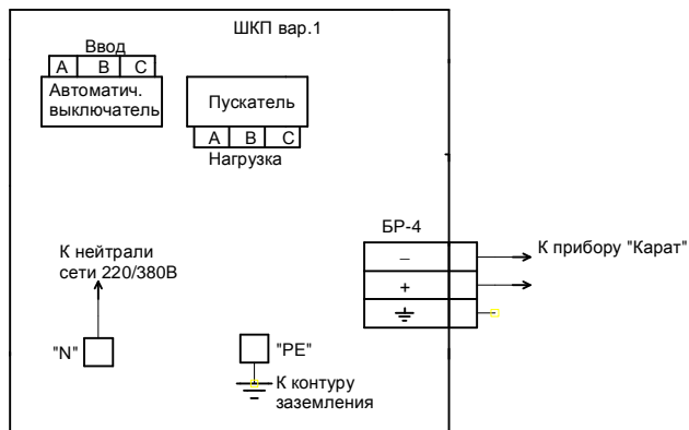
Рис. 1 Схема электрическая подключения шкафов ШКП вар.1
