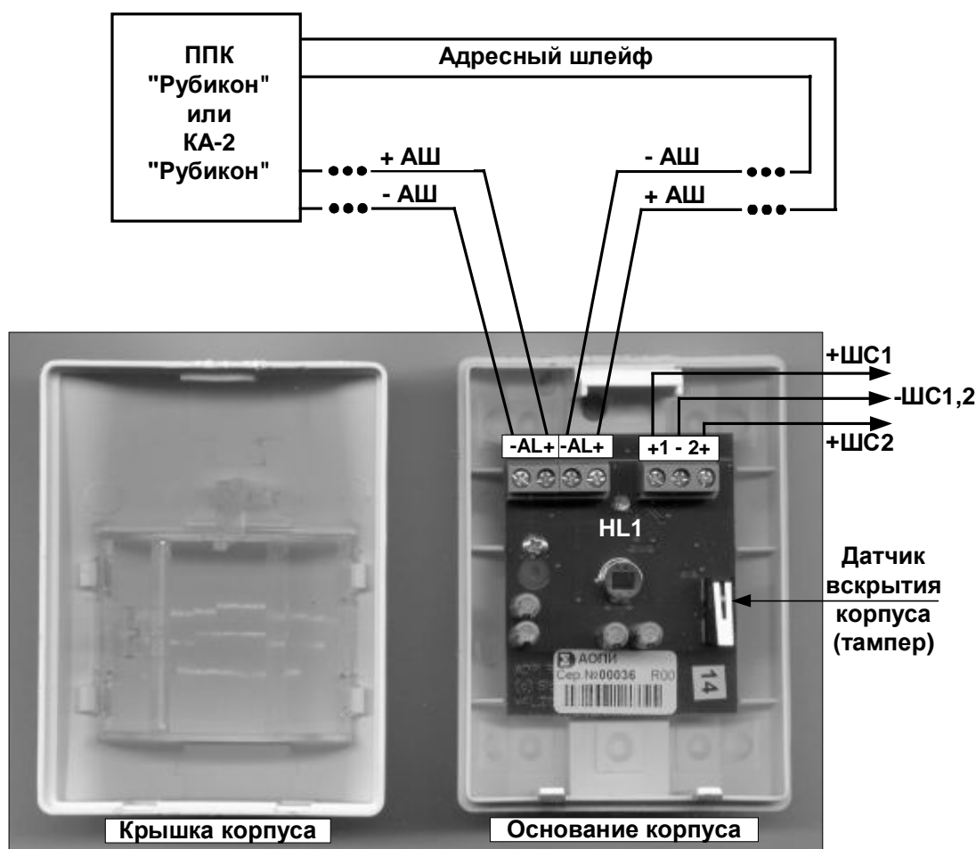
Рис. 2 Конструкция, подключение АОПИ
